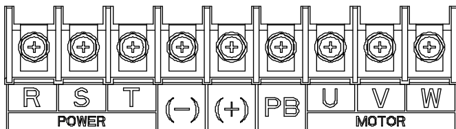
Рис. 4-11 Клеммы силовых цепей 3ф 380В 45–110кВт
