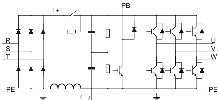
Рис. 3-2 Схема силовой цепи 380В 18.5кВт–110кВт
