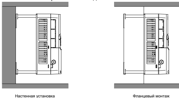
Рис. 4-2 Режим установки
